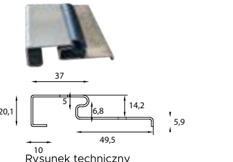
Rysunek techniczny
