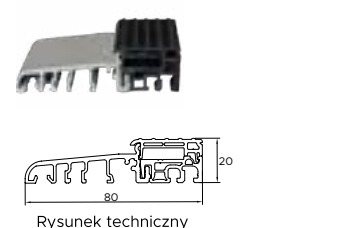
Rysunek techniczny
