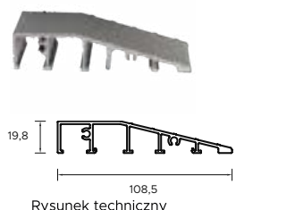
Rysunek techniczny
