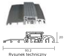
Rysunek techniczny
