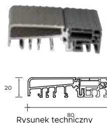
Rysunek techniczny
