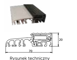
Rysunek techniczny
