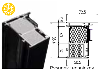
Rysunek techniczny
