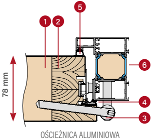
OŚCIEŻNICA ALUMINIOWA
