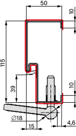
OŚCIEŻNICA STALOWA
