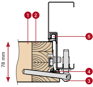
OŚCIEŻNICA STALOWA
