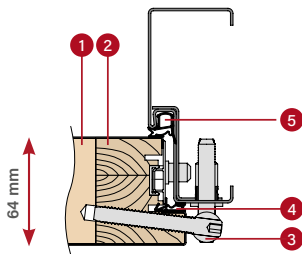
OŚCIEŻNICA STALOWA
