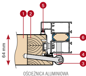
OŚCIEŻNICA ALUMINIOWA
